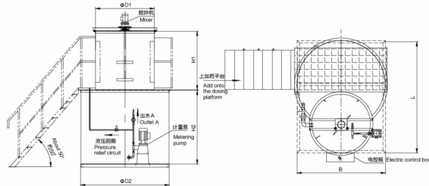
WJY加药装置 WJY Addiction Device
