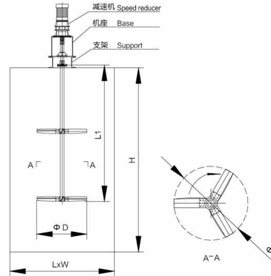
WJB搅拌机图 WJB Mixers
